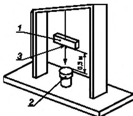
1 — стальная плита; 2 — образец; 3 — стальной прут диаметром приблизительно 38 мм
