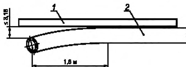
Рисунок D.16 — Измерение концевой прямолинейности
